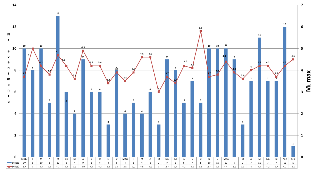
Statistica privind cutremurele vranceane de adancime intermediara ( h > 60\text{km} ) cu M_L \geq 3.0 produse in intervalul 01.01.2017 - 03.09.2019
