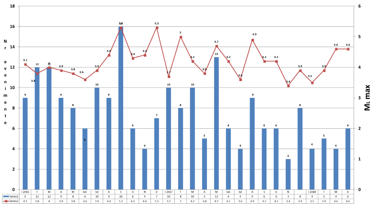
Statistica privind cutremurele vrance de adancime intermediara ( h > 60\text{km} ) cu M_L \geq 3.0 produse in intervalul 01.01.2016 - 25.04.2018
