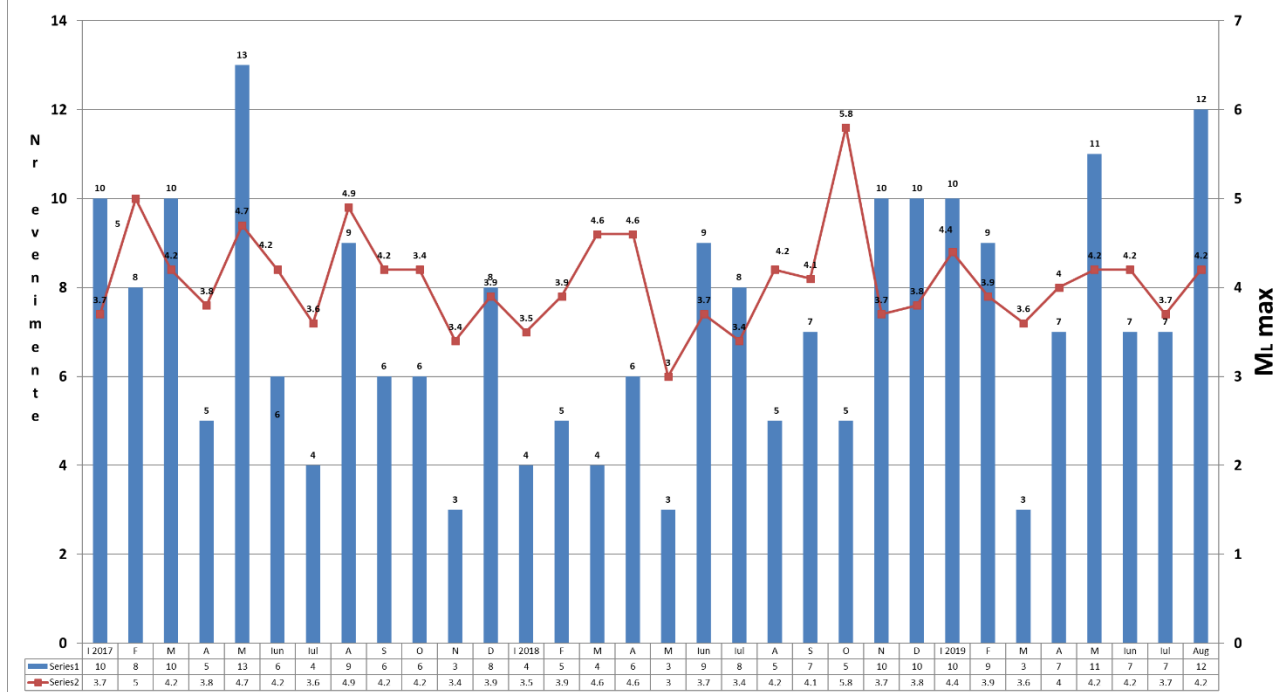
Statistica privind cutremurele vranceane de adancime intermediara ( h > 60\text{km} ) cu M_L \geq 3.0 produse in intervalul 01.01.2017 - 30.08.2019
