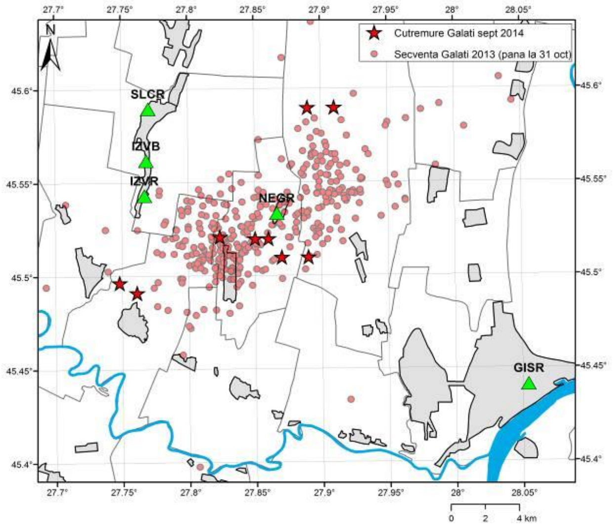
Distributia epicentrelor secventei de cutremure din perioada 10-20 Septembrie 2014
